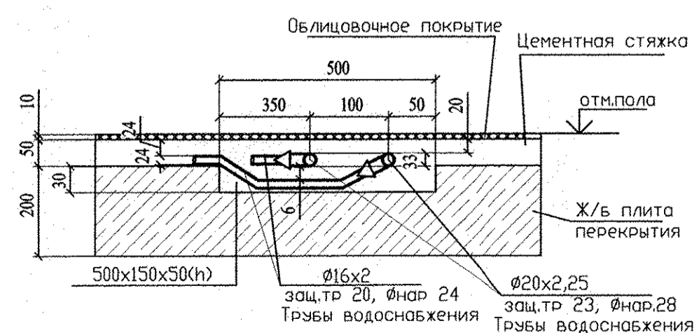
"А" Пересечение труб холодного и горячего водоснабжения
