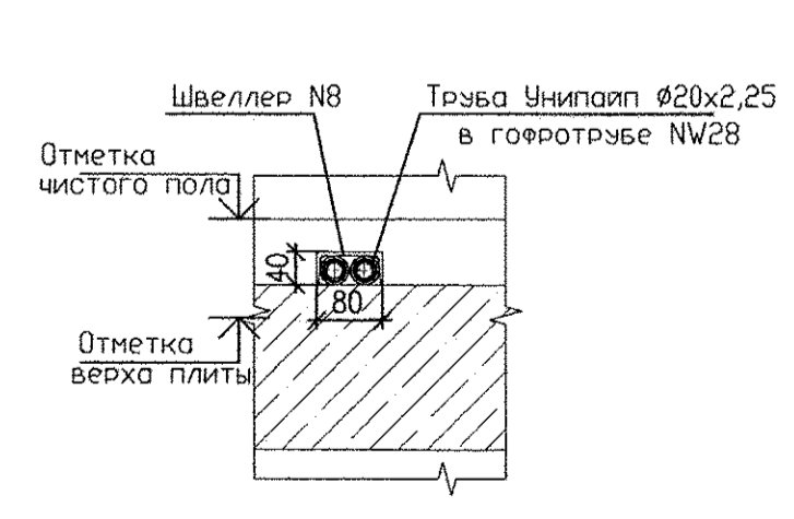
"В" Узел пересечения межкомнатных проемов
